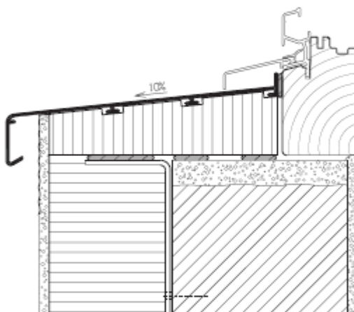
Isolée avec étrier sous Isolation
