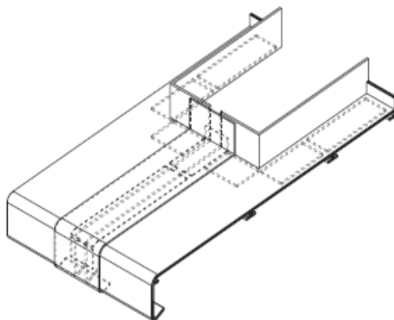
Découpe PB + dilatation
