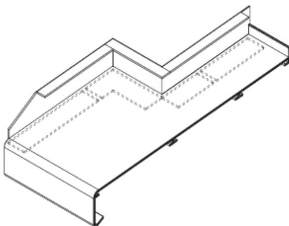
Découpe PC + C
