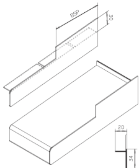
Porte - fenêtre BR - BSP
