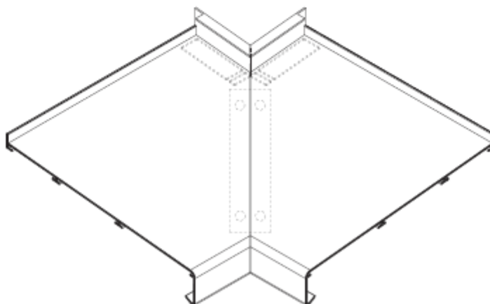
Angle AI - PC
