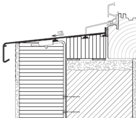
Isolée avec étrier devant Isolation
